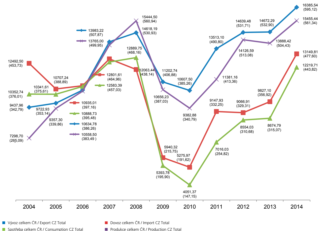
Vývoj vývozu, dovozu, produkce a spotřeby v ČR za období 2004–2014 (HS 8456–8463) v mil. Kč (v mil. EUR) Export, Import, Production and Consumption Development in CZ in 2004–2014 (HS 8456–8463) in mil. CZK (in mil. EUR)
