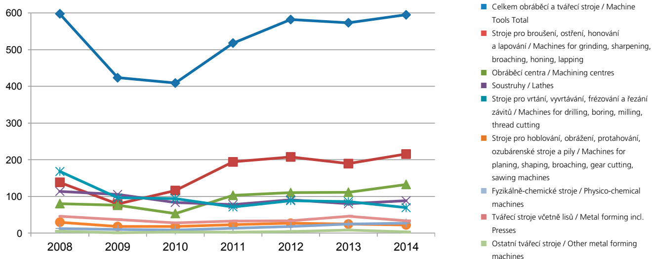
Vývoz obráběcích a tvářecích strojů dle nomenklatur bez ND, příslušenství s GO z ČR v mil. EUR Machine Tool Export acc. to nomenclature without spare parts, accessories, overhauls in mil. EUR
